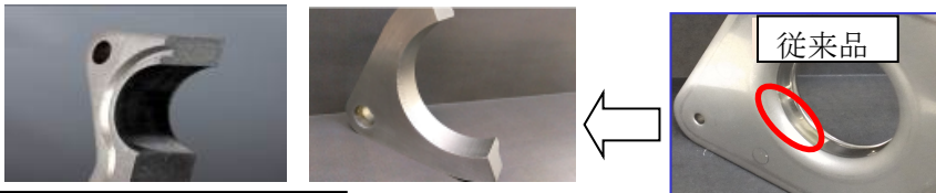
潰し部断面カット図
